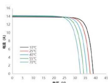
电流-电压曲线 SS8-54HD -410M
